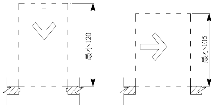
圖 205.2.4.3 無門扇之開口所需之操作空間
