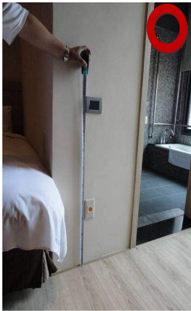
房間內應設置高度90-120公分、 35-45公分共二處求助鈴，以供 輪椅乘坐者求助需求。
