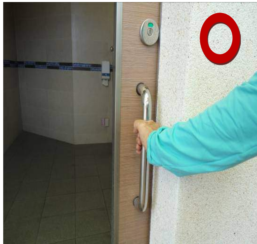
廁所盥洗室應採橫向拉門，出入口淨寬至少80公分，且門把應防止夾手。
