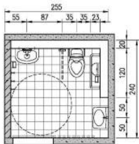
行動不便廁所平立面圖 S=1:50
