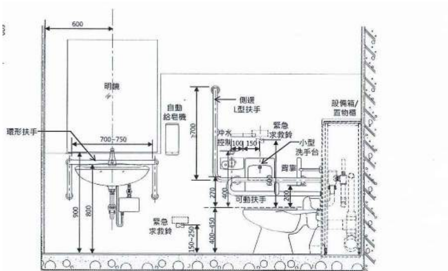
圖2-8a 車站 付費區 無障礙兼性別友善剖面圖
