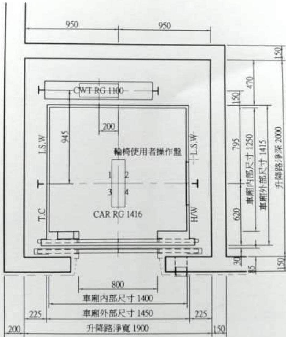
電梯間平面圖
